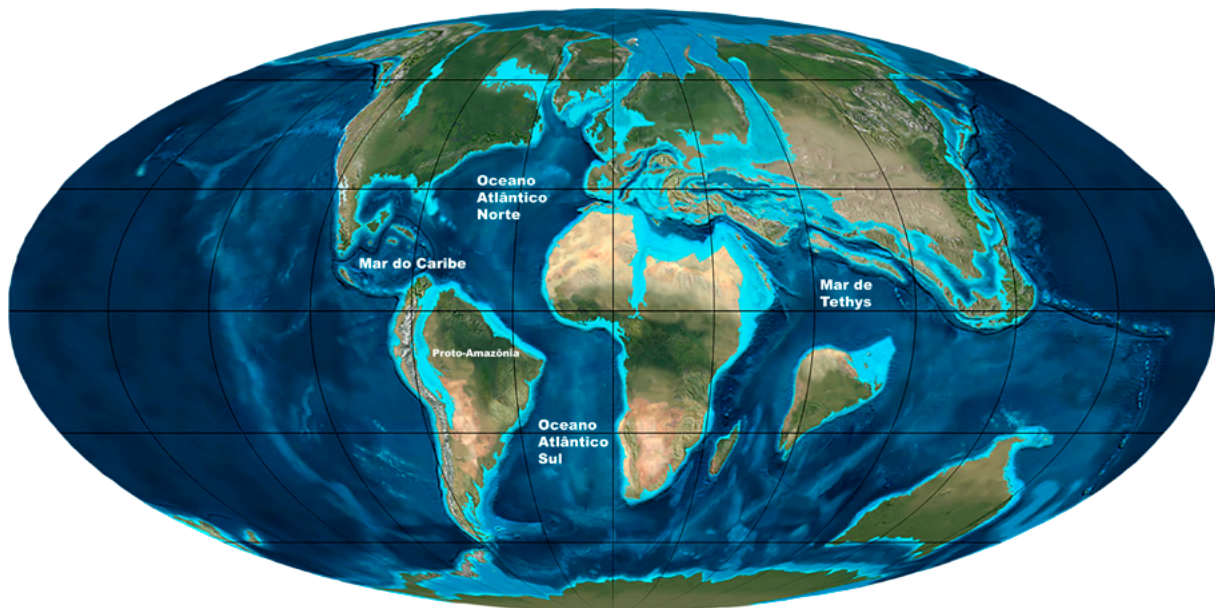
Figura 3: Reconstrução paleogeográfica da Terra durante o final do Período Cretáceo e a passagem para o Paleógeno (cerca de 66 milhões de anos). Estão indicados os principais mares e oceanos, além da Região Proto-Amazônia. Fonte: modificado de Ron Blakey Deep Time Maps™ (deeptimemaps.com) (2019).
