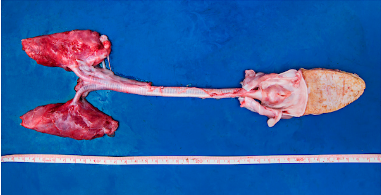
Figura 19: Língua e Sistema respiratório de um espécime de Caiman latirostris . Foto: Leonardo Merçon.
